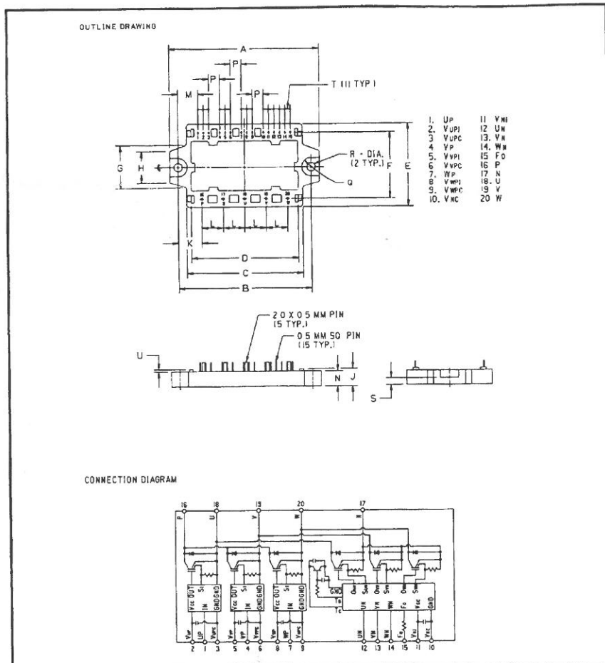
110-230 Volt Line, PM20CHA060 Outline Drawing
