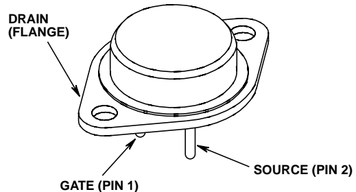
JEDEC TO-204AE
